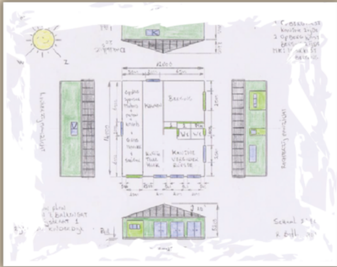
Een eerste schets van het speeltuingebouw, uitgewerkt in een voorlopig ontwerp
